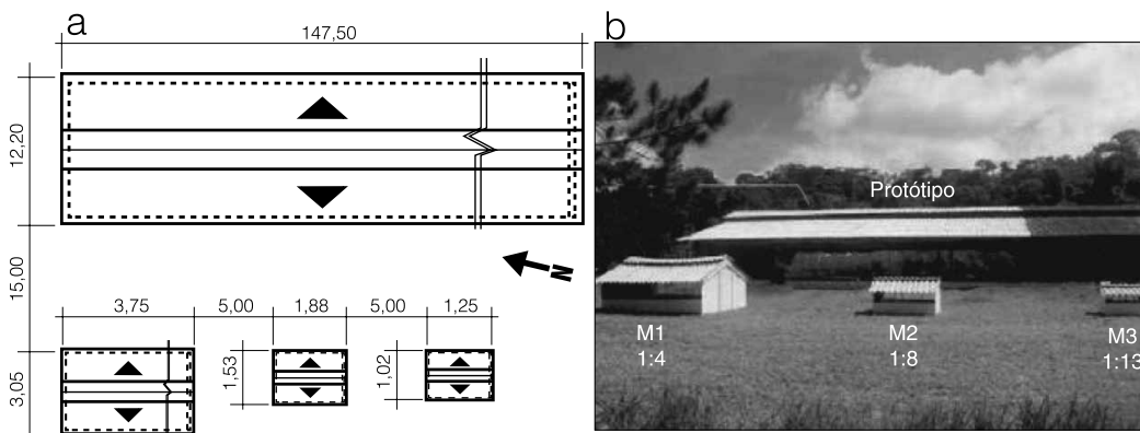
Figura 2. Esquema ilustrativo da disposição dos tratamentos em campo (a) e vista da extremidade do protótipo e dos modelos reduzidos em campo (b).
