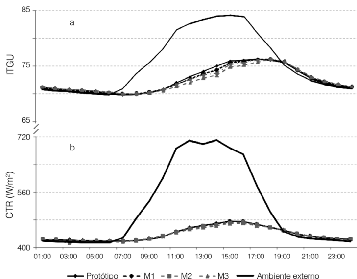
Figura 3. Médias do índice de temperatura do globo negro e umidade (ITGU) e carga térmica de radiação (CTR, em W\ m^{-2} ), correspondente ao nível das aves, em função dos horários de medição no interior do protótipo e dos modelos físicos reduzidos avaliados e no ambiente externo.
